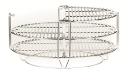
"Divide & Conquer"
